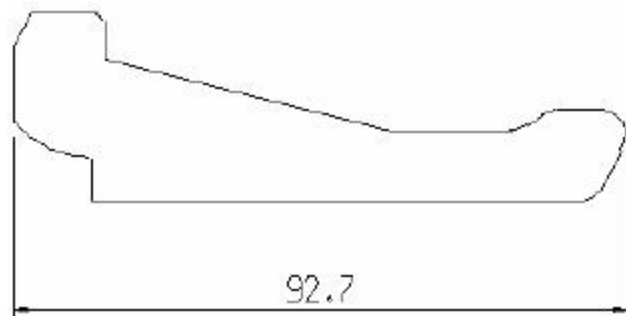
G9/004 Spannfinger AS100 347-10-2130/000 100621
