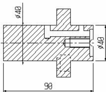
G9/035P Bolzen Zentralblock
