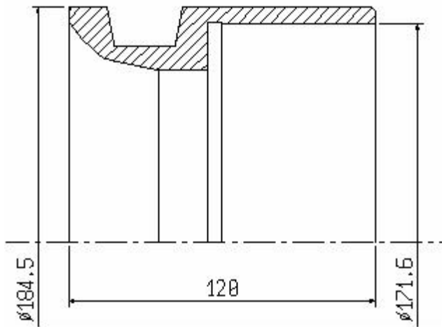
G9/001 Spannmuffe AS82
