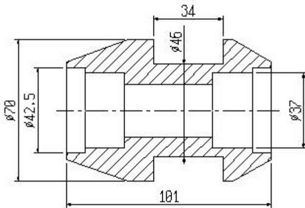
G9/050A Rolle
