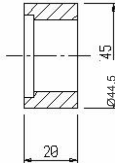
G9/030R Rolle 305-08-1420
