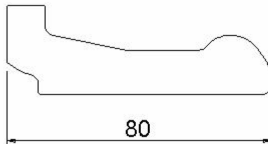
G14/003 Spannfinger 703-10-0017/000 100620
