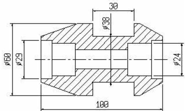
G9/050B Rolle
