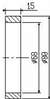
S4/008B Pierścień docisku 383
