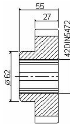
S5/059 Z40 Koło zębate SD50d688b
