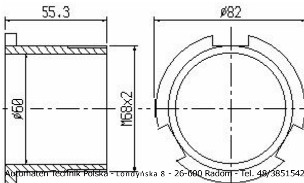
S4/007A Tuleja 372
