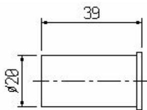
S5/036P Ośka
