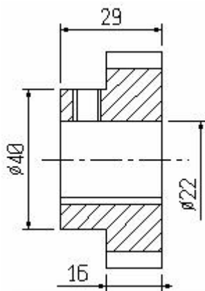
S5/058 Z23 Koło zębate SD63d1069
