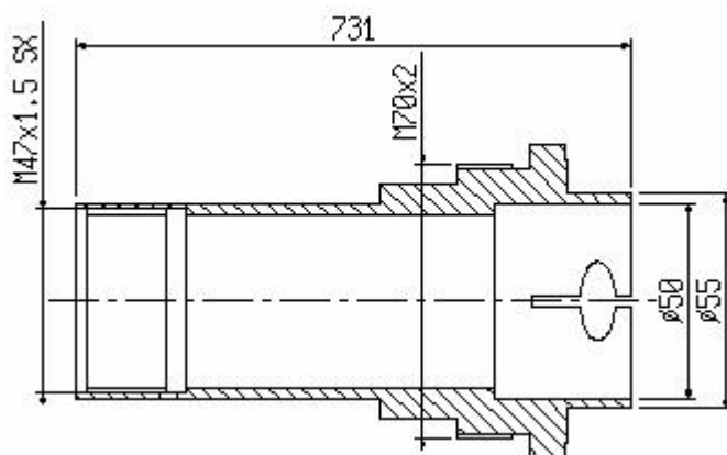
S4/010 Rura zacisku 341
