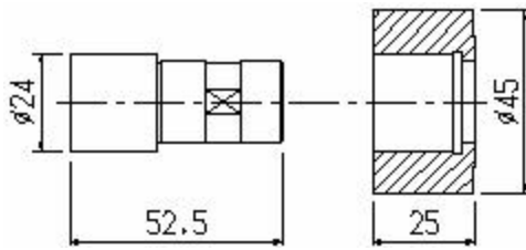
S5/030P (186) Oś
