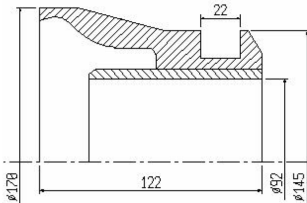
S5/001 Mufa zacisku SD50c376
