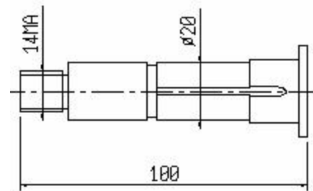
S5/034P Ośka
