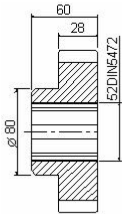
S5/061 Z39 Koło zębate SD50d689a
