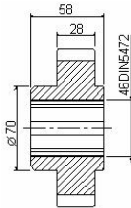
S5/060 Z51 Koło zębate SD50d690a
