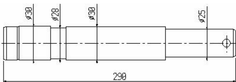
S4/056 Wał
