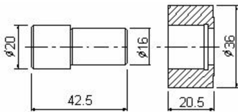
S4/030P Ośka
