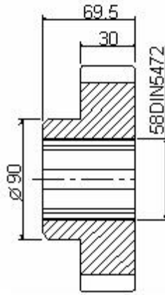
S7/054 Z52 Koło zębate 685
