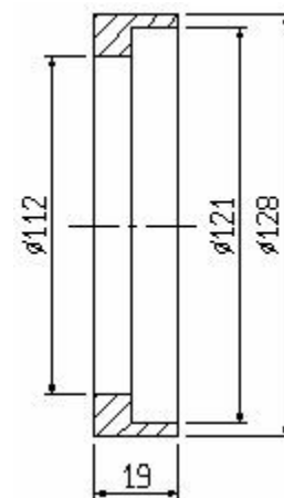
S4/011 Pierścień
