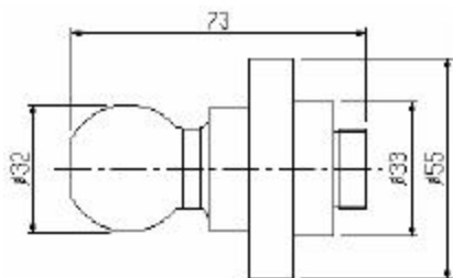
S5/039 Kulowy bolec M20x1,5
