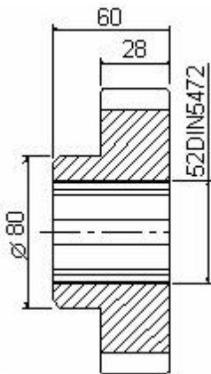
S5/063 Z46 Koło zębate SD50d685a
