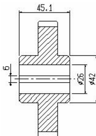
S4/057 Koło zębate Z50 VD32d744A
