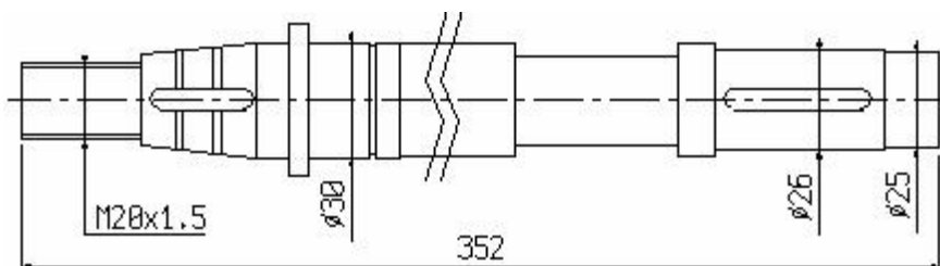
S4/058 Wał SD63d121a
