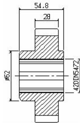
S5/052 Z40 Koło zębate 706
