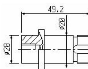
S7/030P (612) Oś
