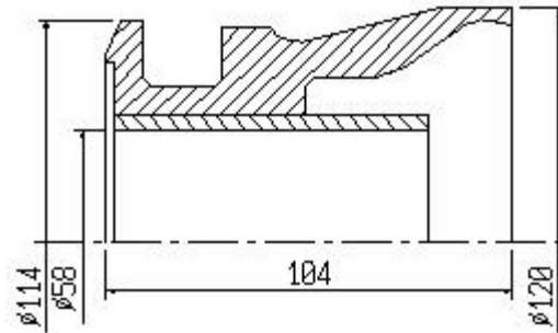
S4/001B mufa zacisku SD25 376+329
